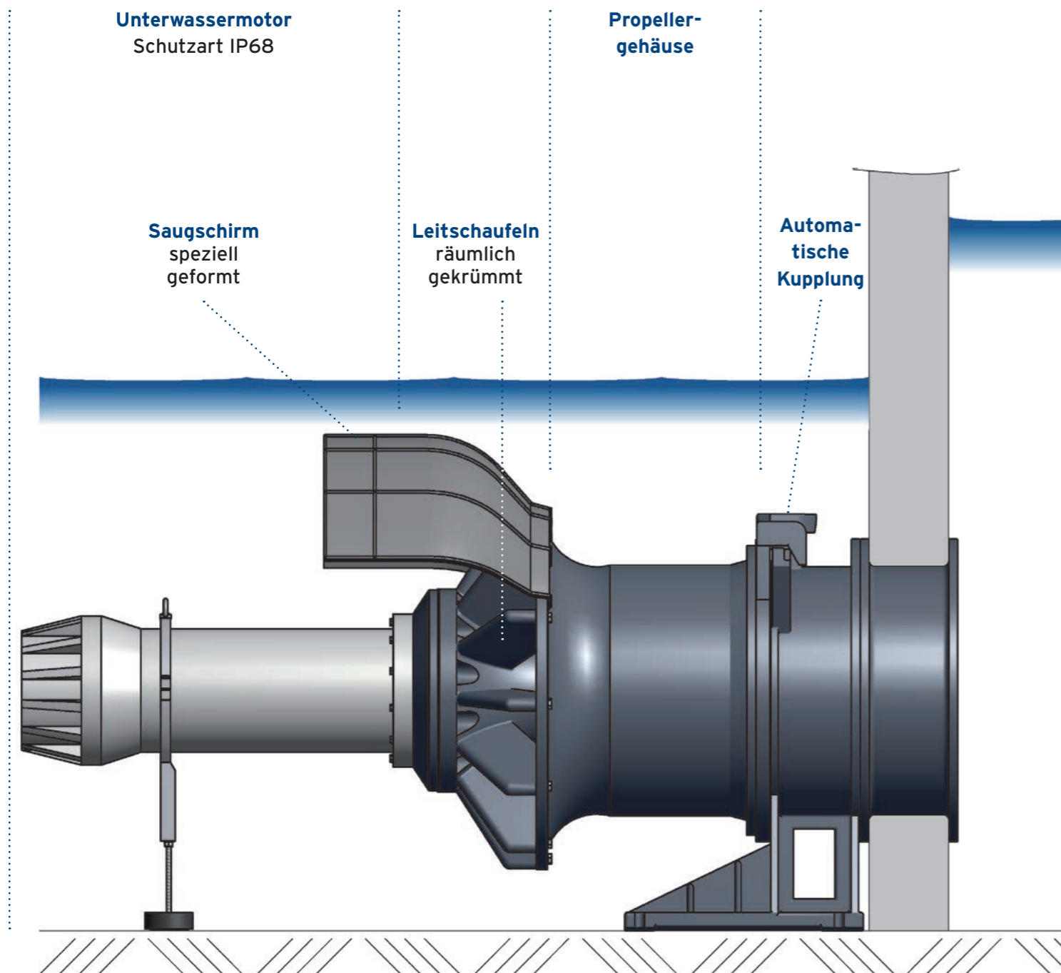
Horizontale Tauchmotor-Propellerpumpe HUP 600
