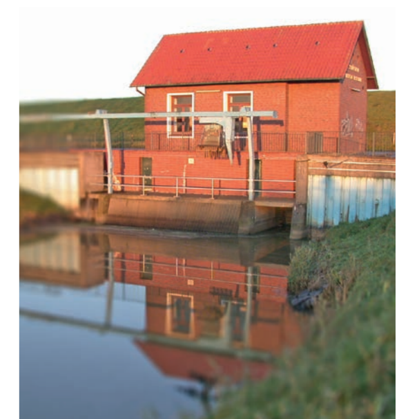
Schöpfwerk Haselau VP 1000 Vertikale Propellerpumpe 3.400 l/s 5,0m 250 kW
