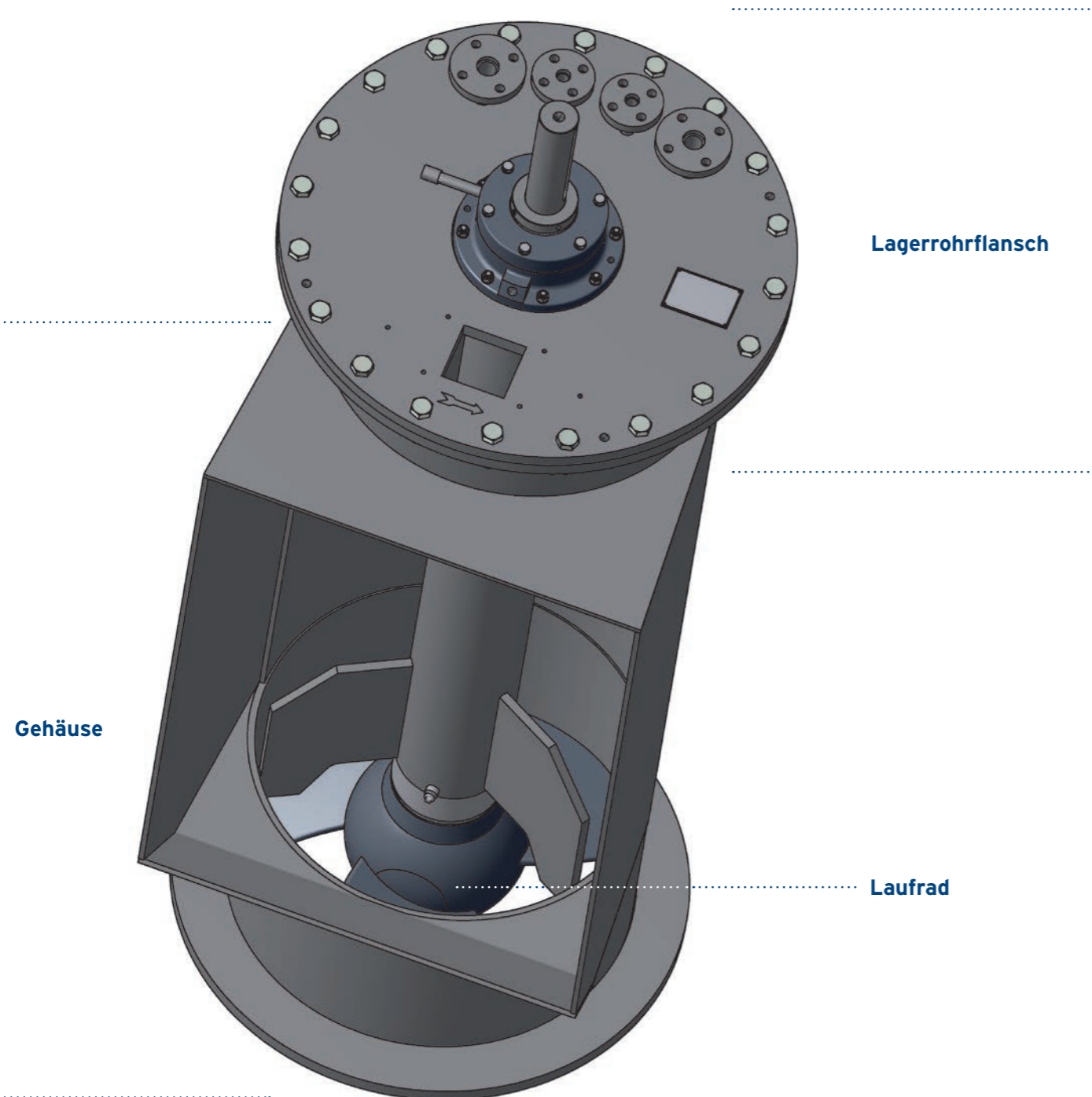
Umwälzpropellerpumpe UWP 600 (Darstellung ohne Motor)
