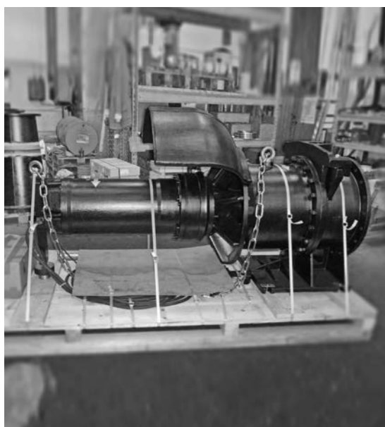
Schöpfwerk Aalbeek Siel HUP 600 Horizontale Tauchmotorpumpe 1.200 l/s 3,0m 55 kW
