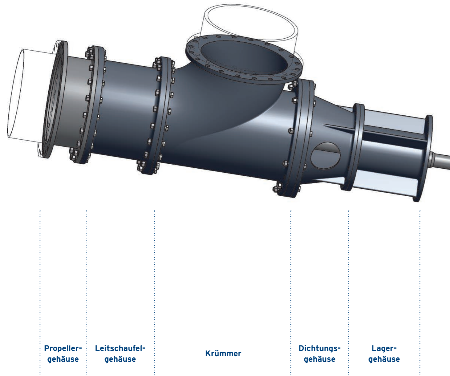
Inline-Bogenpumpe IBP 500 (Darstellung ohne Motor)
